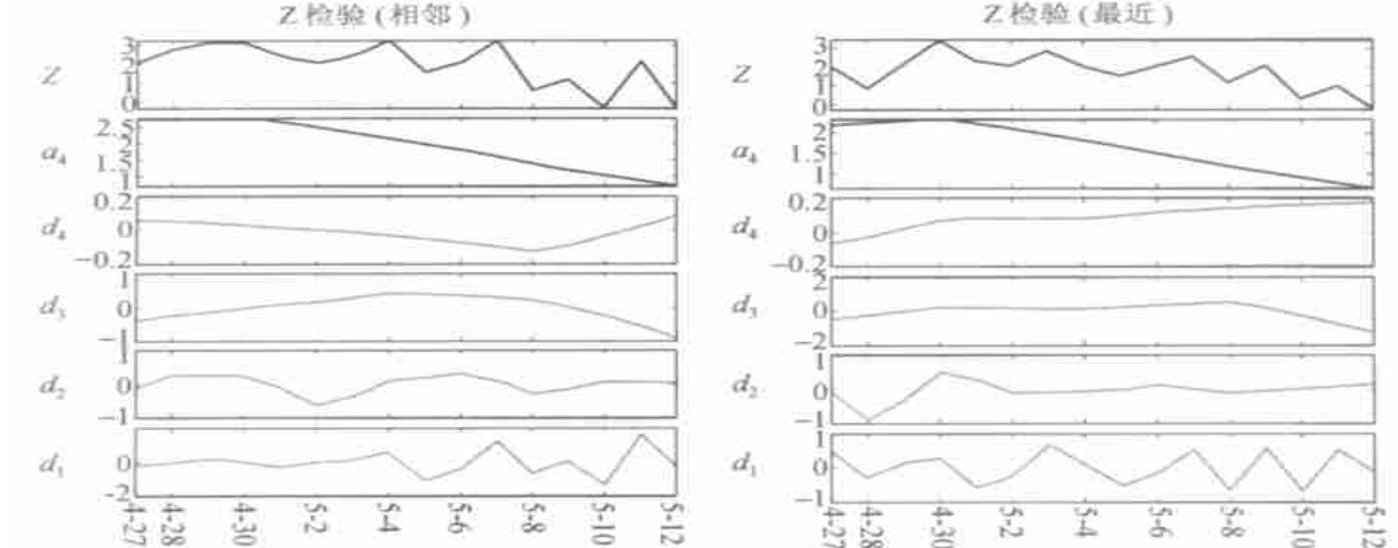
图 10 北京 18 区 SARS 新增病例 BW 检验频谱分解
